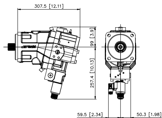
Regolatore RPS RPS Control
